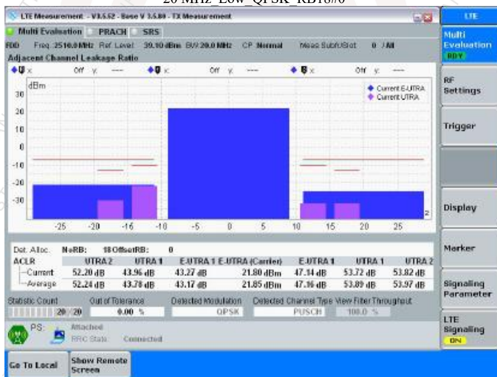
20 MHz Low QPSK RB18#0
